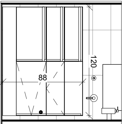
חדית למשטח כיור לארון תנור 2 1 : 25
