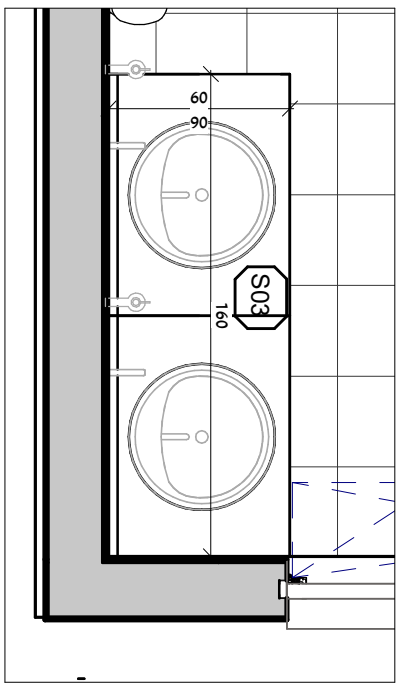
מעטת ניורים שירותי מטופלים 1 1 : 25
