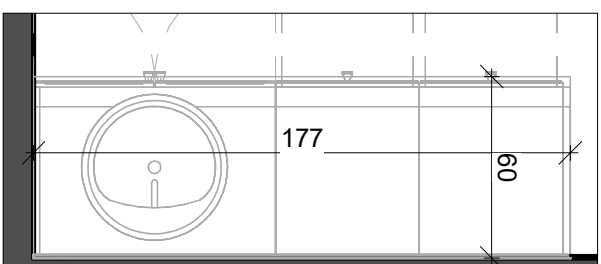
משטח כיוור לארון חדר טיפול 1 1 : 25
