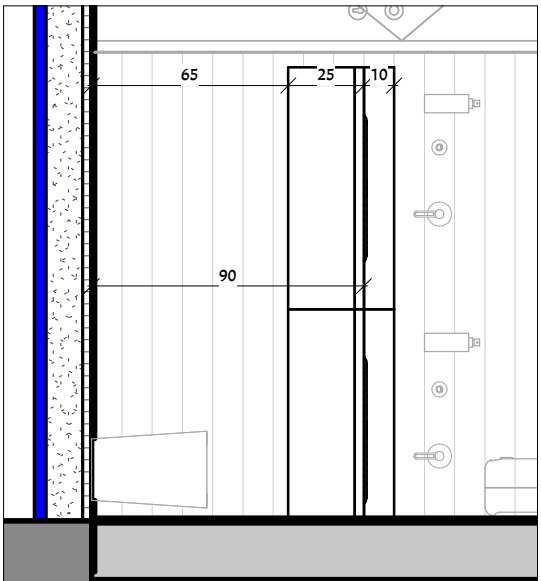
S02 2 1 : 25
