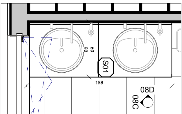
משטח ניורים שירותי צוות נשים 1 : 25 1
