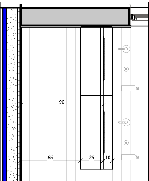
S01 1 : 25 2
