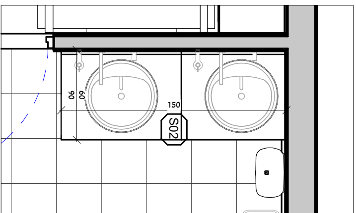
משטח כיורים שירותי צוות גברים 1 1 : 25
